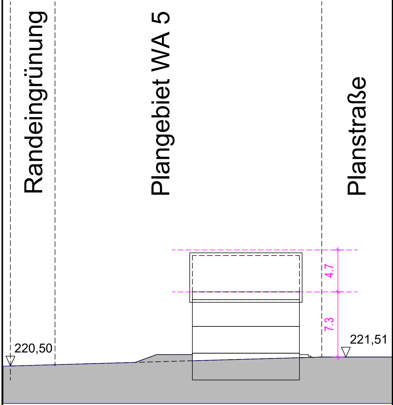
Geländeschnitt C-C
