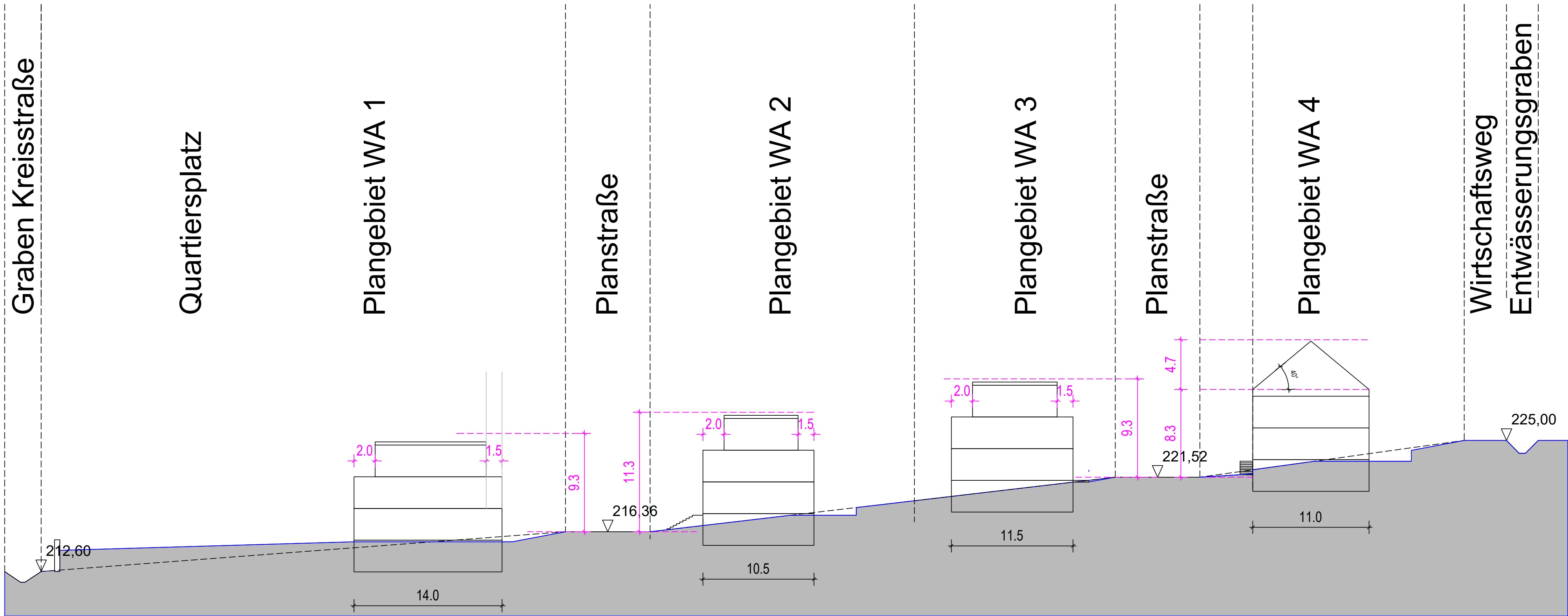
Geländeschnitt B-B
