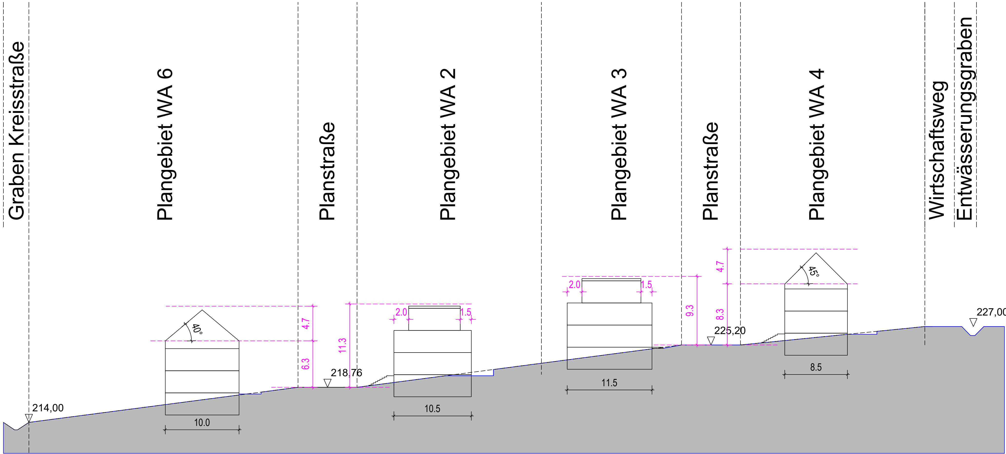
Geländeschnitt A-A
