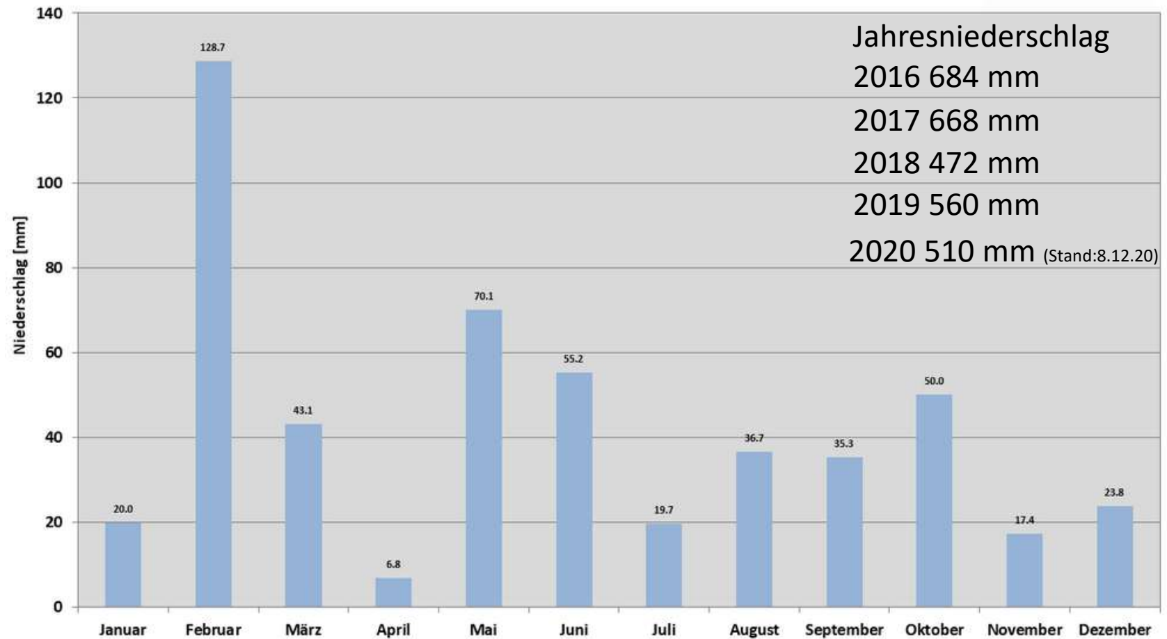
Monatssumme des Niederschlags - Groß-Umstadt 2020
